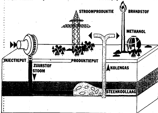
Schematische voorstelling van een ondergrondse kolenvergassingsproject.
